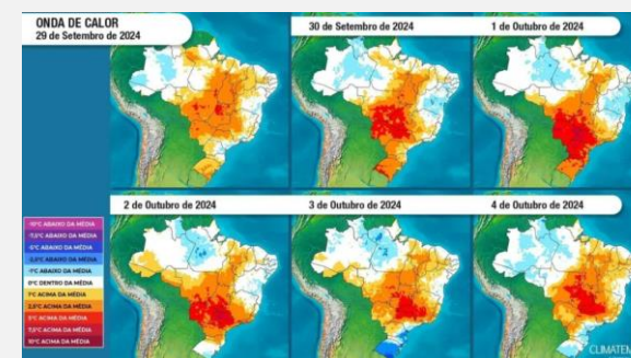
Evolução da onda de calor no Brasil entre 29.09.2024 e 04.10.2024
